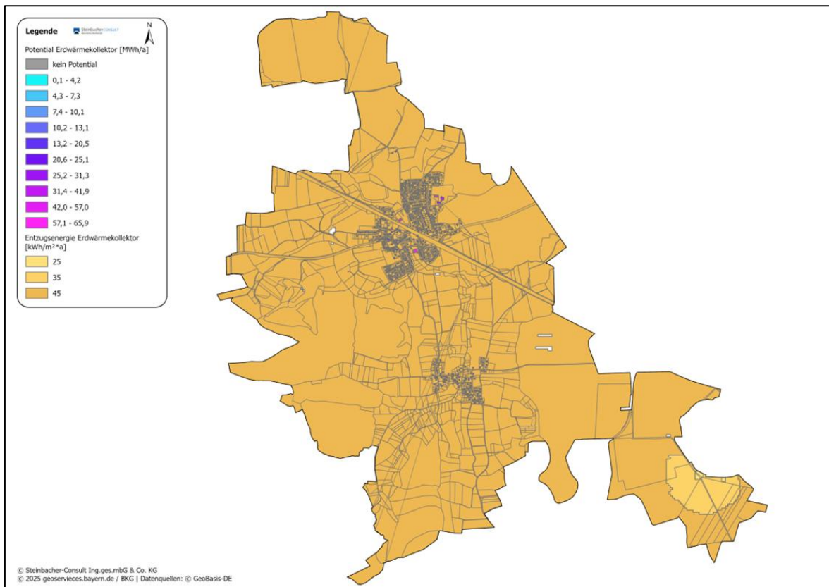
Abbildung 16: Entzugsenergie Erdkolektoren
