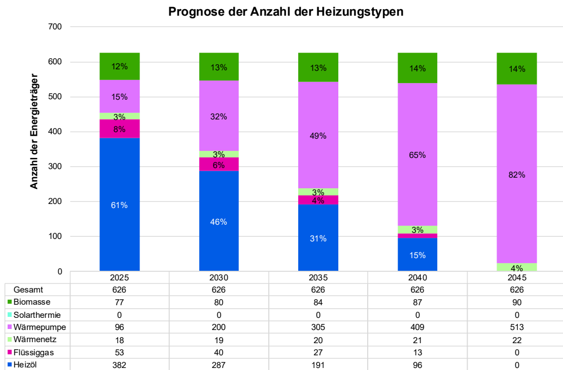
Abbildung 27: Entwicklung Wärmeerzeuger
