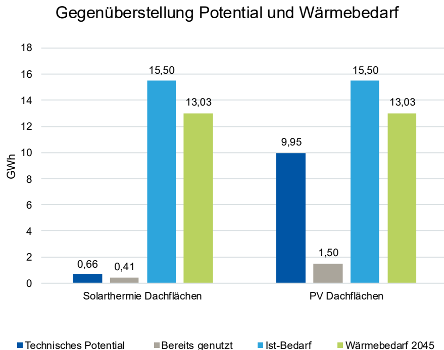
Abbildung 15: Dachflächenpotenzial
